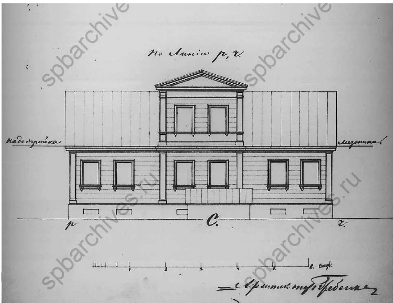
Чертеж особняка до и после перестройки в 1906 году
